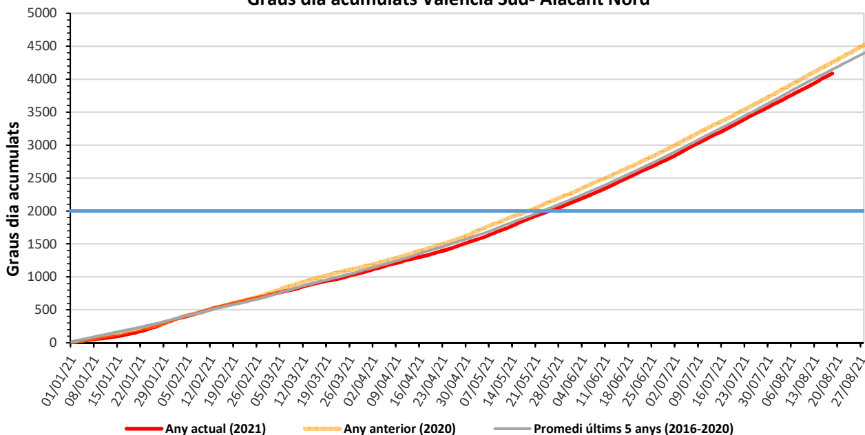
Graus dia acumulats València Sud- Alacant Nord
